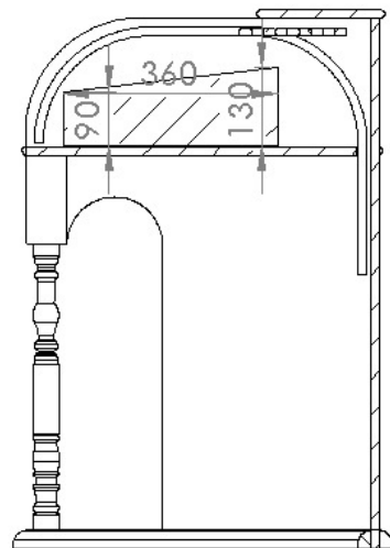
SEÇÃO A-A ESCALA 1 : 13
